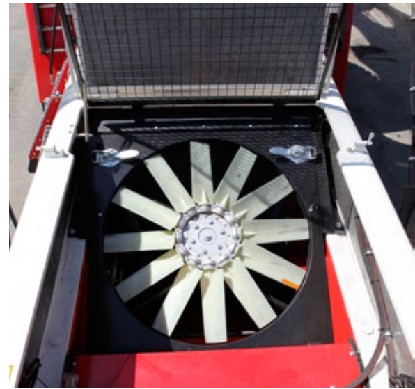
Reversible hydrostatic fan
